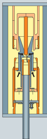
Выключение: дуогасительный контакт в разомкнутом положении
