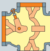
Заземлитель в замкнутом положении
