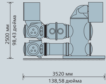
Ячейка кабеля
