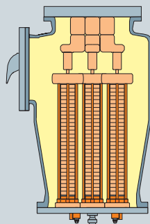
Ограничитель перенапряжений нелинейный
