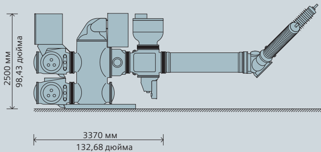
Модуль прямого подключения трансформатора
