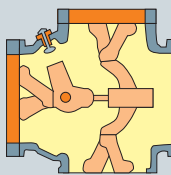
Разъединитель в замкнутом положении
