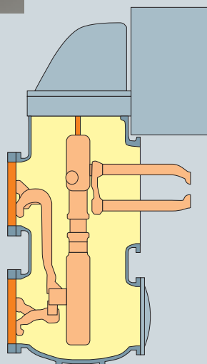
Силовой выключатель
