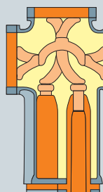
Пример: модуль непосредственного подключения кабеля (традиционного типа)
