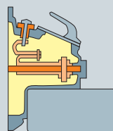
Быстродействующий заземлитель
